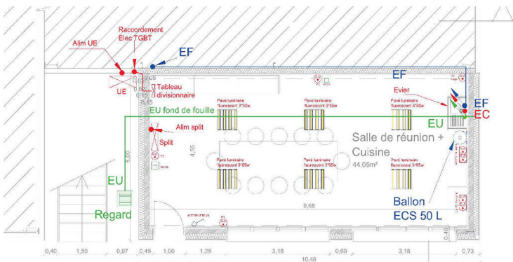
Plan du RDC extension PROJET
