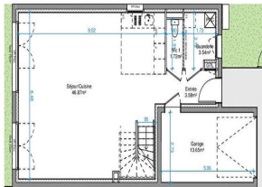
- PLAN RDC -
